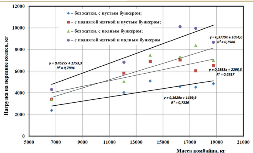
Рис. 2. Нагрузка на переднее колесо комбайнов в технологическом процессе комбайнирования
