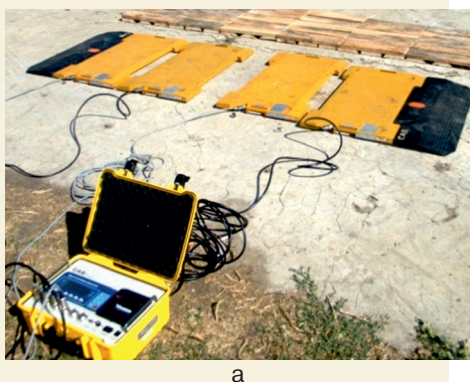
Рис. 1. Тензометрические весы (а) и схема приложения сил к комбайну ДОН-1500Б в различных комплектациях (б)
