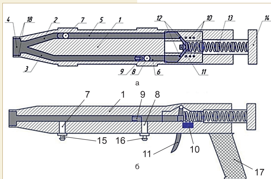
Рис. 1. Универсальный пистолет-распылитель (сопло) для формирования распыла жидкого материала грунтовок: а – вид сверху; б – вид сбоку
