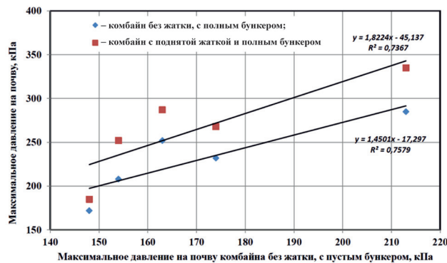
Рис. 4. Зависимость максимального давления колес исследуемых комбайнов на почву по вариантам их производственного применения от базовых показателей
